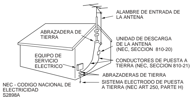
EjemPlo de conEXion a tierra de la antena segun el código nacional de electricidad
